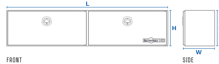
HD DOUBLE DOOR TOP MOUNT
