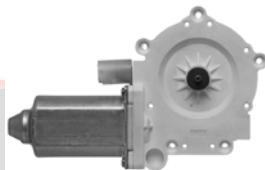
88041 B88041 ACI Plus Power Window Motor Mini (05-02) BMW: 67626955875 Mini: 67626955875
